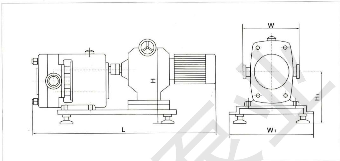
主要参数和外形尺寸 Main Parameters and Overall Dimensions
