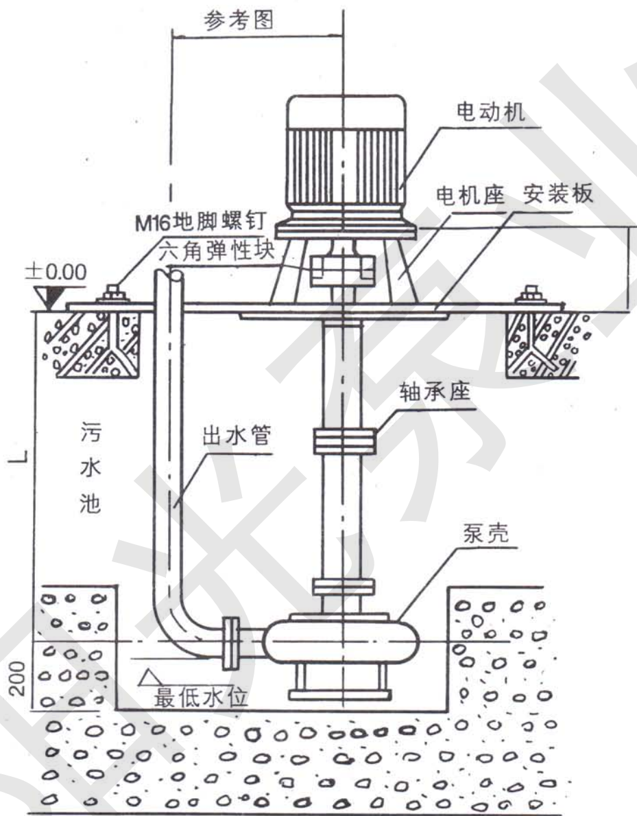
污水泵固定安装示意图
