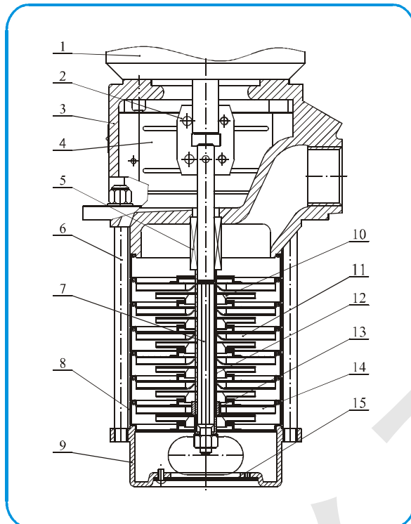
截面图 CDLK,CDLKF8,16,20
