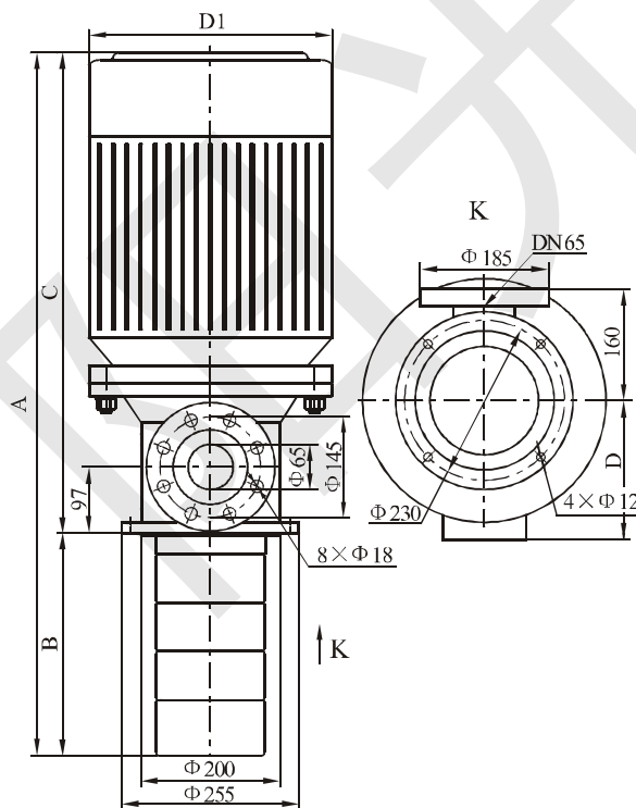
安装图
