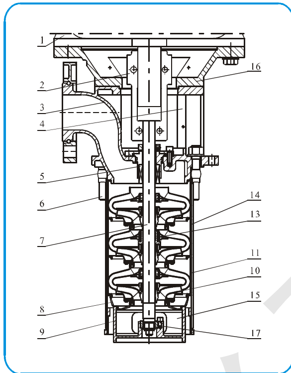
截面图 CDLK,CDLK F32,42
