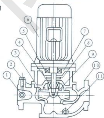
热水型结构
