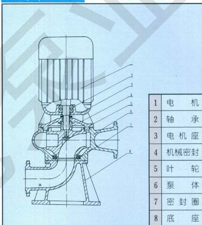
LW(I)型结构
