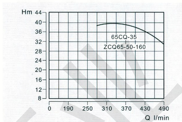
磁力泵性能曲线图(以常温清水为测试介质)
